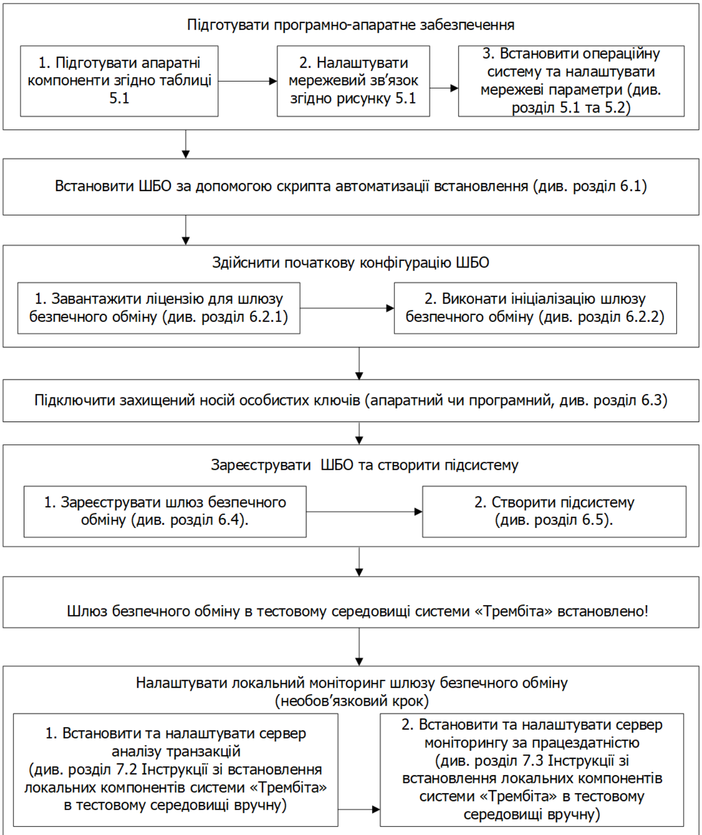
Рисунок 4.1 – Блок-схема алгоритму встановлення локальних компонентів системи «Трембіта» в тестовому середовищі вручну
