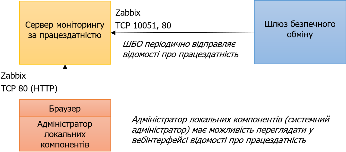
Рисунок 7.2 – Схема мережевої взаємодії сервера моніторингу за працездатністю
