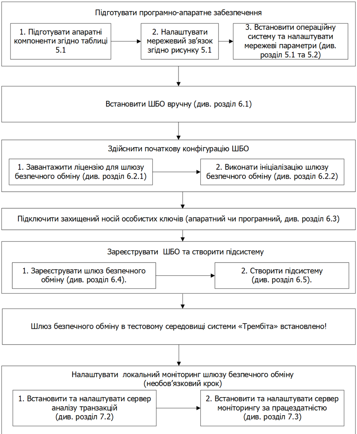
Рисунок 4.1 – Блок-схема алгоритму встановлення локальних компонентів системи «Трембіта» в тестовому середовищі вручну
