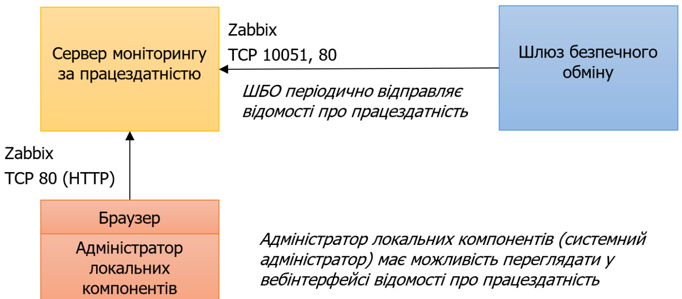
Рисунок 7.2 – Схема мережевої взаємодії сервера моніторингу за працездатністю
