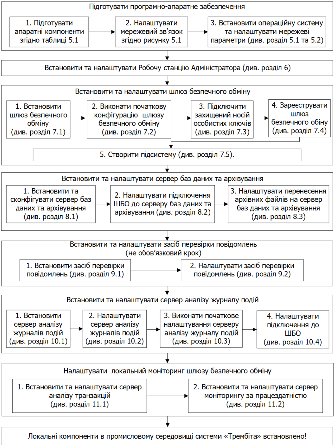
Рисунок 4.1 – Блок-схема алгоритму встановлення локальних компонентів системи «Трембіта» в промисловому середовищі
