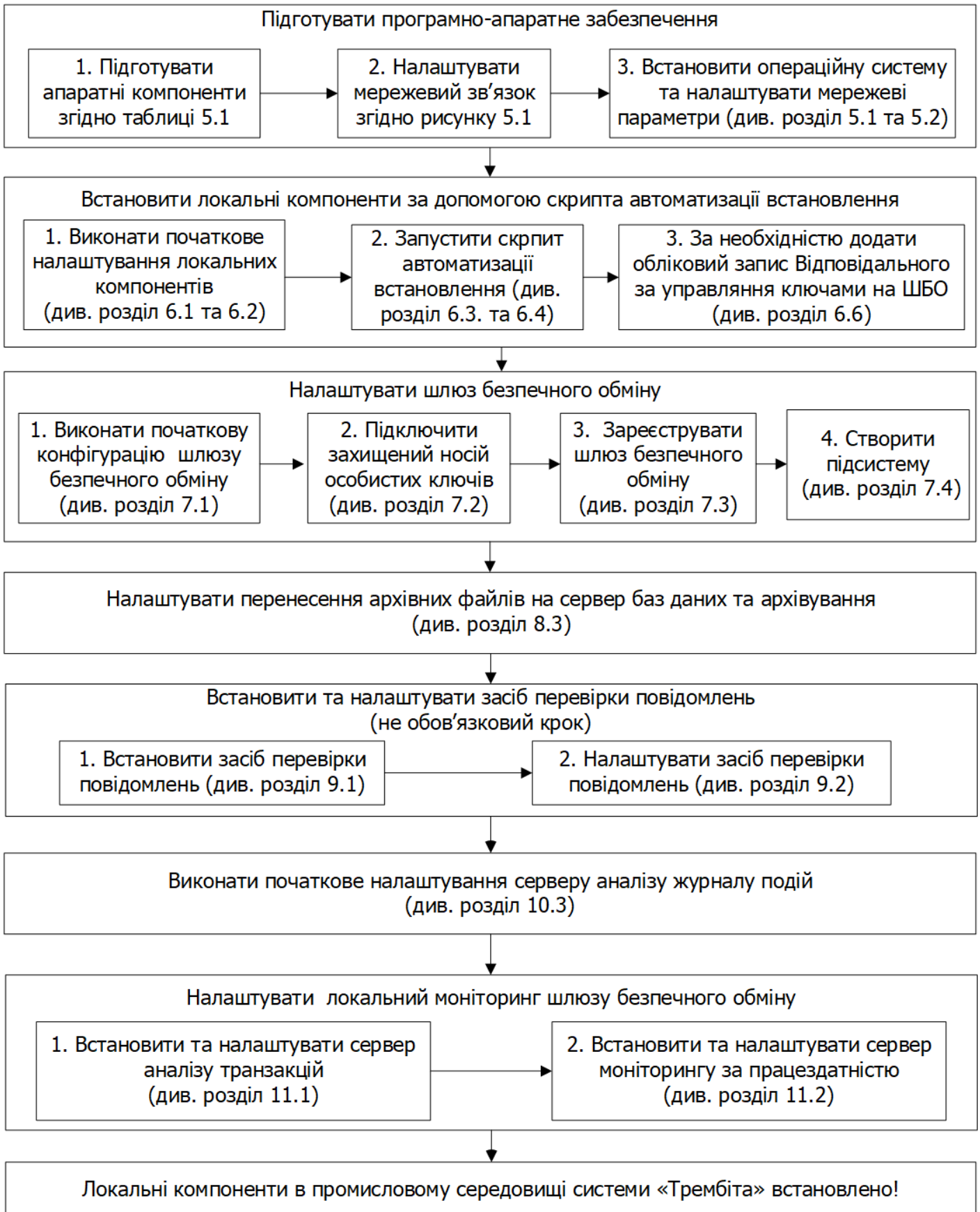
Рисунок 4.1 – Блок-схема алгоритму встановлення локальних компонентів системи «Трембіта» в промисловому середовищі вручну
